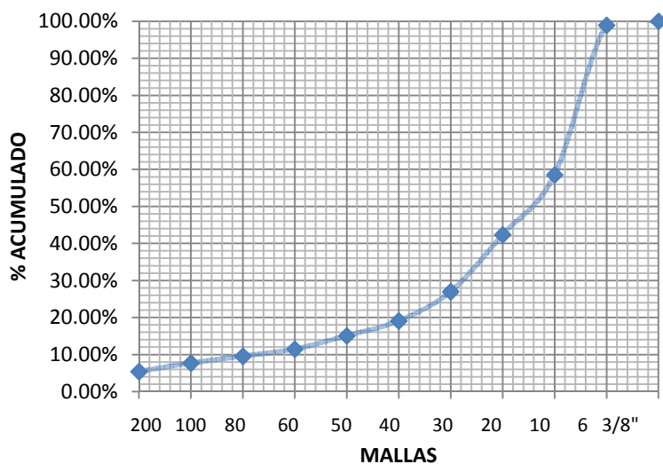
CURVA GRANULOMETRICA
